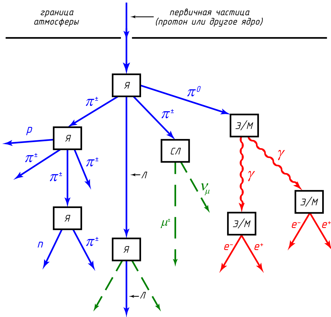
Рисунок 3. Качественная схема взаимодействия протона космических лучей с ядрами в земной атмосфере: Л — лидирующая частица; Я — ядерное взаимодействие; Э/М — электромагнитное; СЛ — слабое.
