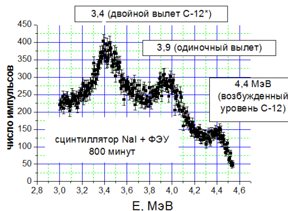
рис.4.3. Фрагмент спектра мгновенных \gamma -квантов, снятый сцинтилляционным спектрометром с кристаллом NaI(Tl) 40*40 мм. Сравните с Вашим спектром.
