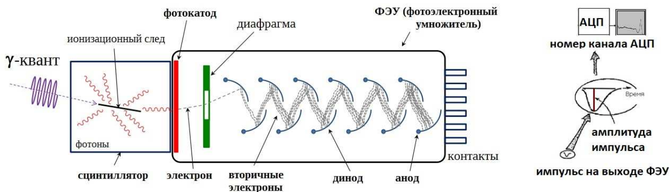
Рис. 5.1: Схема устройства сцинтилляционного детектора. Частица, попадая в сцинтиллятор, порождает фотоны флюоресценции, которые по светопроводу попадают на фотокатод ФЭУ. По амплитуде выходного импульса с ФЭУ на АЦП добавляется «единичка» в соответствующий номер канала
