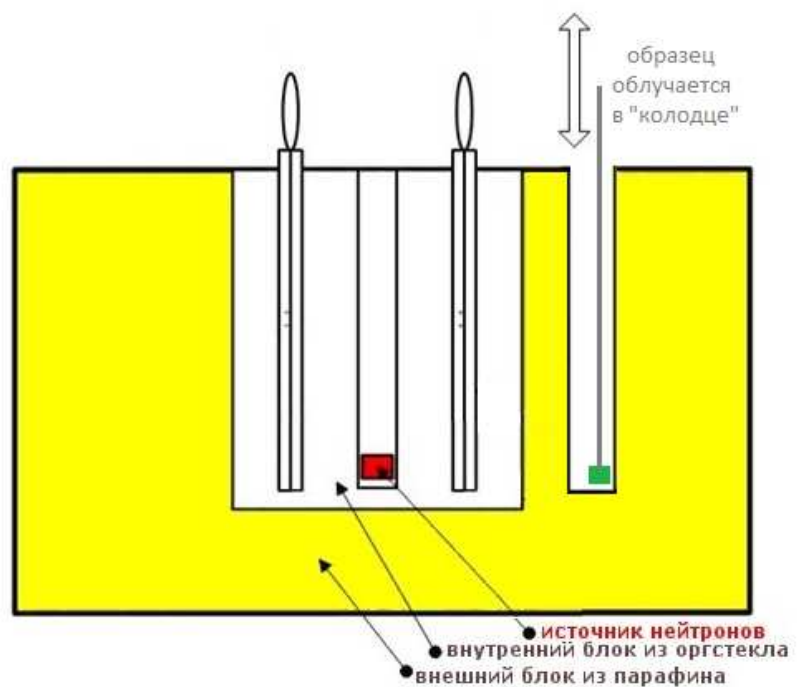
рис.4.2. Схема активации образцов
