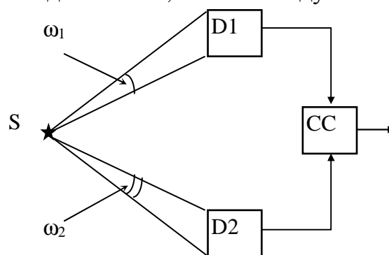
Рис. 3. Схема установки двойных совпадений: S – радиоактивный источник, D1 и D2 – детекторы, СС – схема совпадений.
