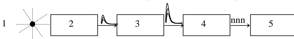
Рис. П1. Блок-схема спектрометра
