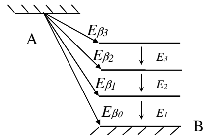
Рис. 5. \beta -распад ядра А в ядро В с несколькими парциальными \beta -спектрами.
