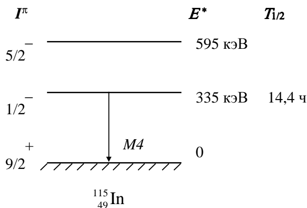
Рис. 1. Схема нижних уровней ядра ^{115}_{49}\text{In} .
