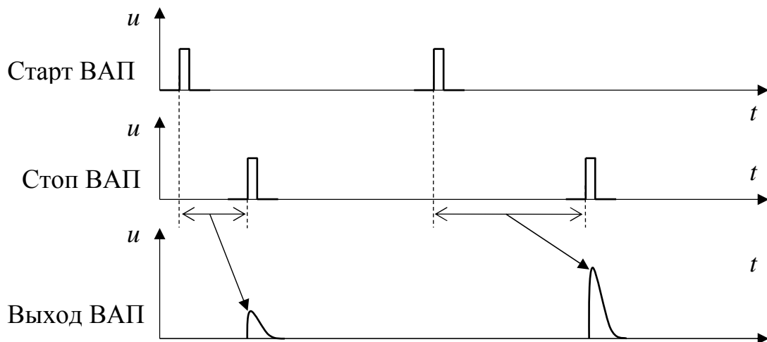
Рис 6. Сигналы на входах и выходах ВАП
