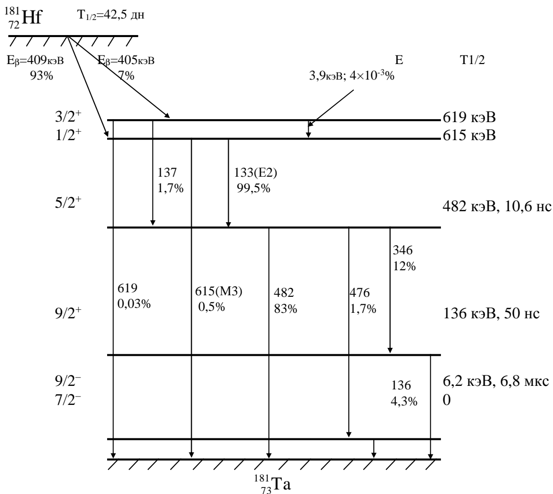
Рис. 2. Схема распада ^{181}_{72}\text{Hf} (приведены только основные \gamma -переходы).
