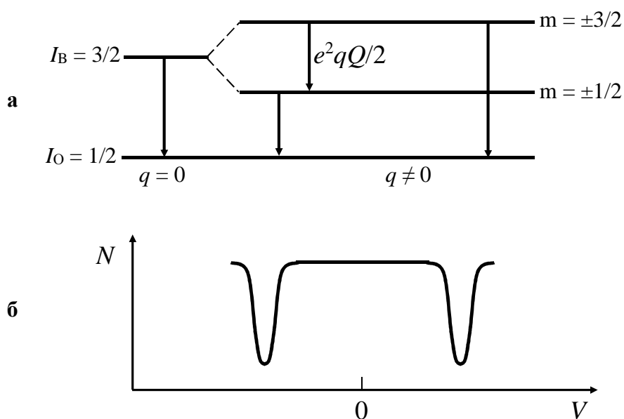
Рис. 7. Переходы между подуровнями возбужденного состояния с I_B = 3/2 и основным состоянием ( I_0 = 1/2 ) – (а) и вид мессбауэровского распределения – (б) для случая квадрупольного сверхтонкого взаимодействия. Схема подуровней возбужденного состояния соответствует e^2 q Q > 0 .
