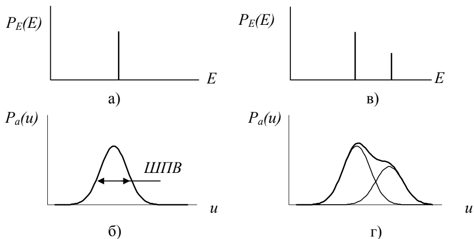
Рис.2. Энергетический спектр и амплитудное распределение: а) монохромный спектр (синглет), б) амплитудное распределение одиночной линии, в) две близкие линии (дублет), г) амплитудное распределение дублета.
