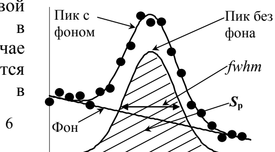
Рис. 6. Результат аппроксимации пика.
