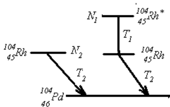
Рис. 19. Схема распада ^{104}_{45}\text{Rh} и ^{104}_{45}\text{Rh}^*
